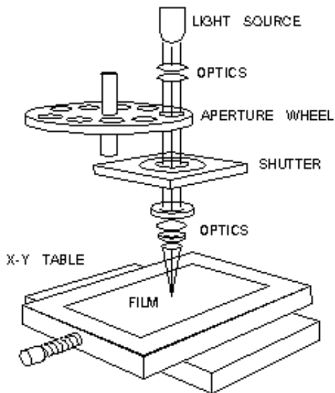
Rys 1 - Schemat działania fotoplota
