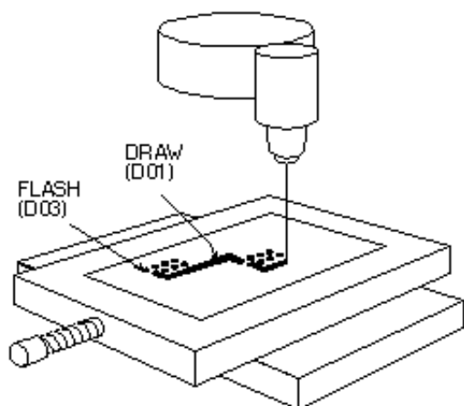
Rys 2 - Praca plotera
